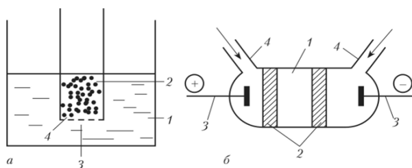
Рис. 7.11. Схемы диализа (а) и электродиализа (б):
